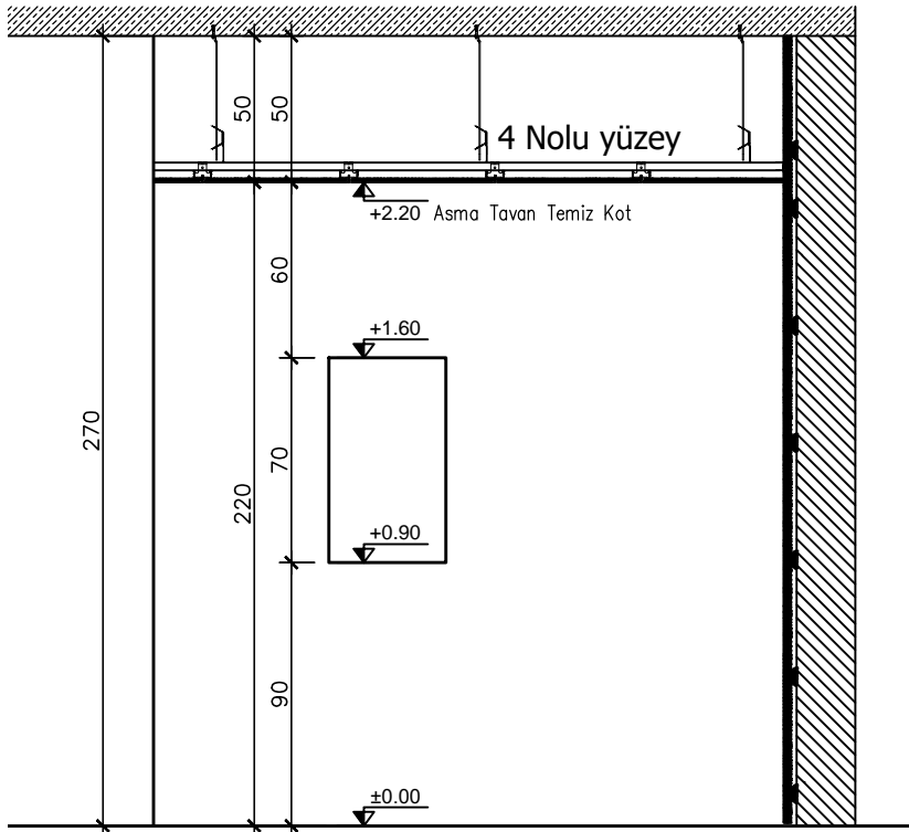
A-A KESİTİ
