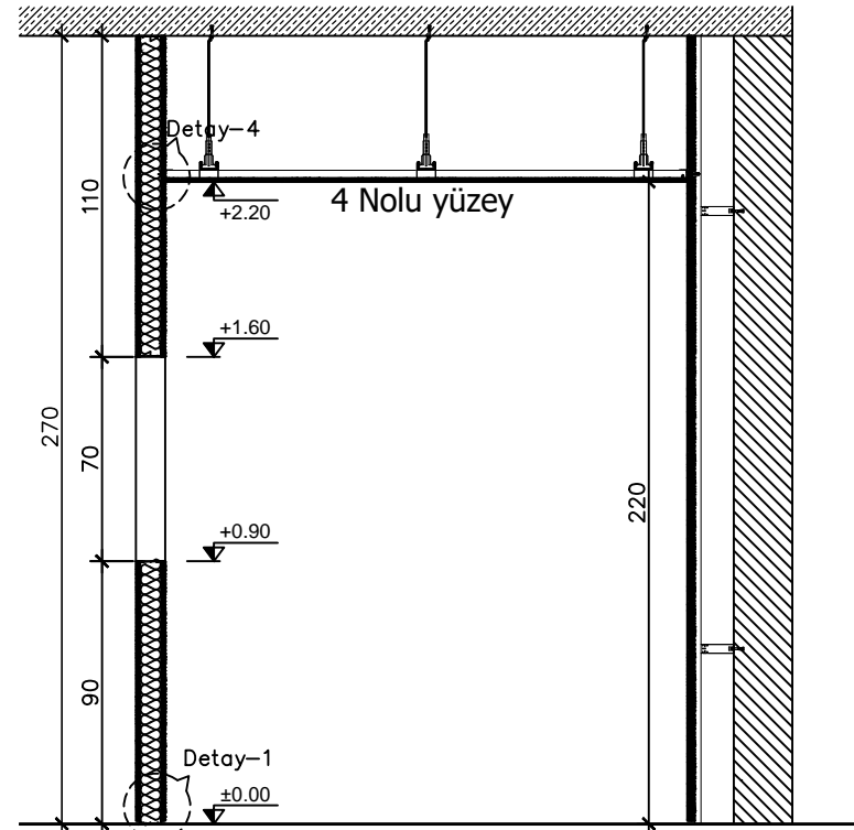
B-B KESİTİ
