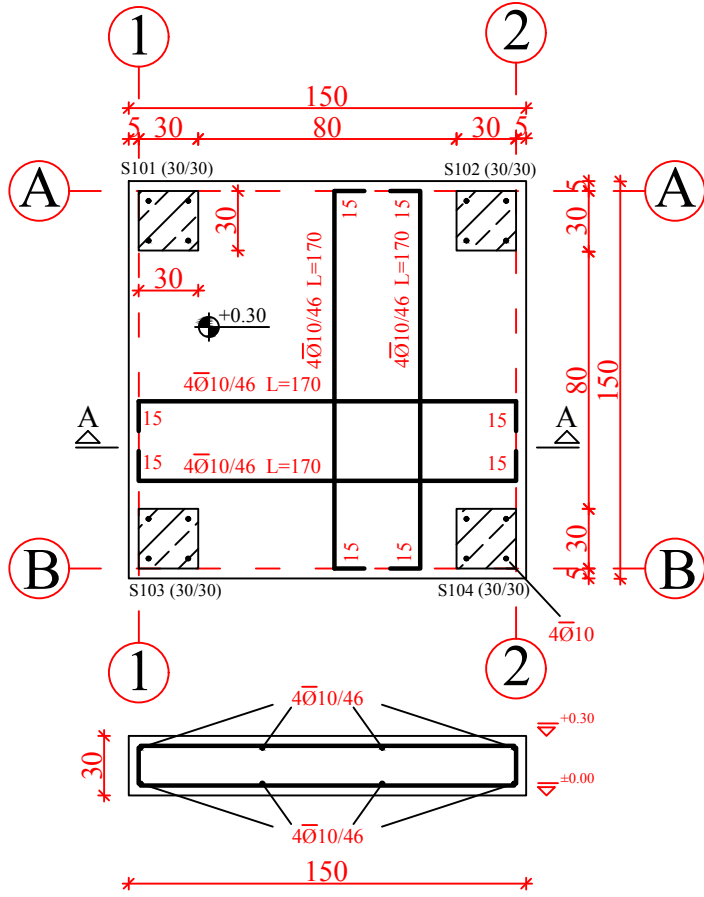
KESİT A-A
